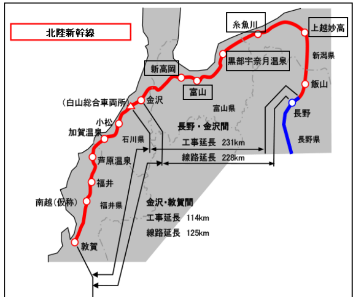
上図:北陸新幹線概要図 (鉄道建設・運輸施設整備支援機構HPより)
