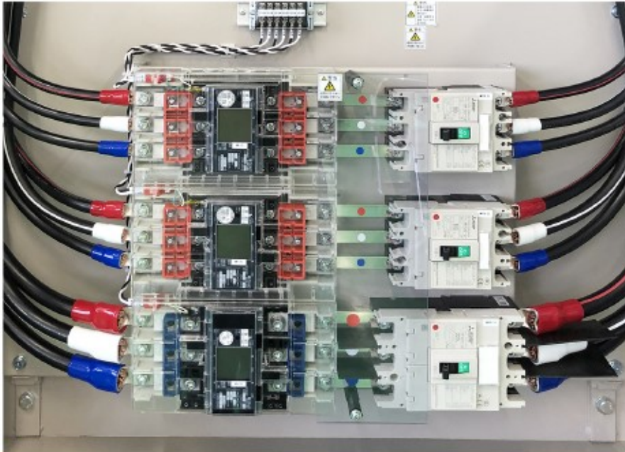
設置状況
